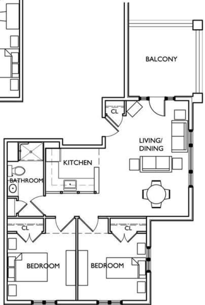
2 BEDRM TYPE A
